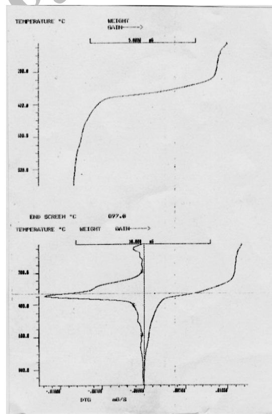
تصویر ۷. نمودار DTG نمونه شاهد که پیک پیرولیز سلولز در 345^{\circ}\text{C} رخ می‌دهد.
