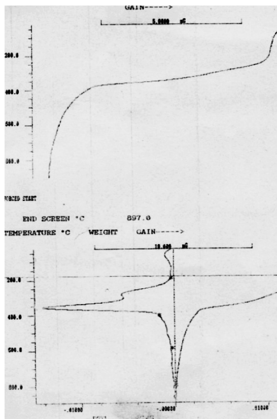
تصویر ۸. نمودار DTG نمونه درمان شده با محلول هیدروکسید باریم که نمونه یک پییک پیرولیز در دمای 344^{\circ}\text{C} دارد (با یک اختلاف دمای 6/8^{\circ}\text{C} ) نسبت به نمونه شاهد
